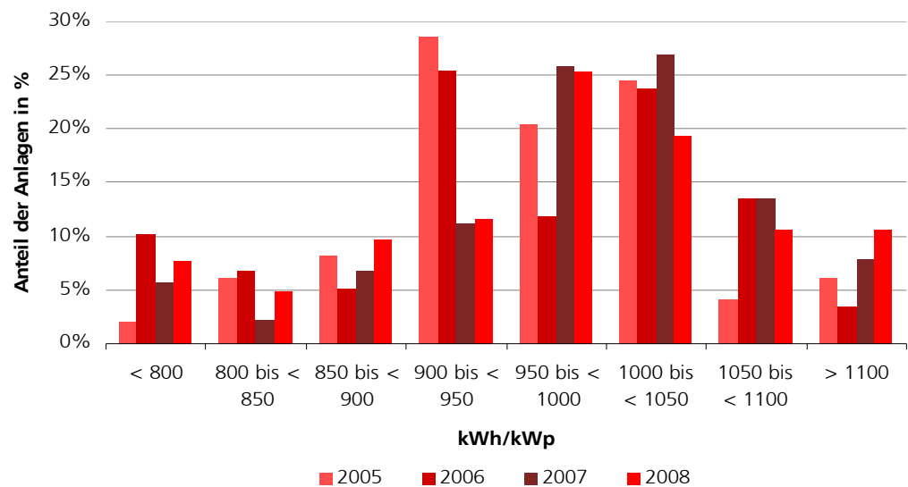
Bild 1: Verteilung des Jahresertrages sämtlicher Anlagen für die Jahre 2005 bis 2008
