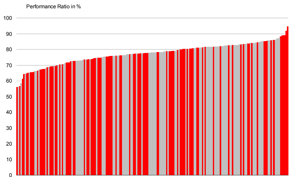
Bild 3: 100 Anlagen in Süddeutschland aus dem ISE- Monitoring (grau) im Vergleich mit den Anlagen des Powerchecks (rot) .
