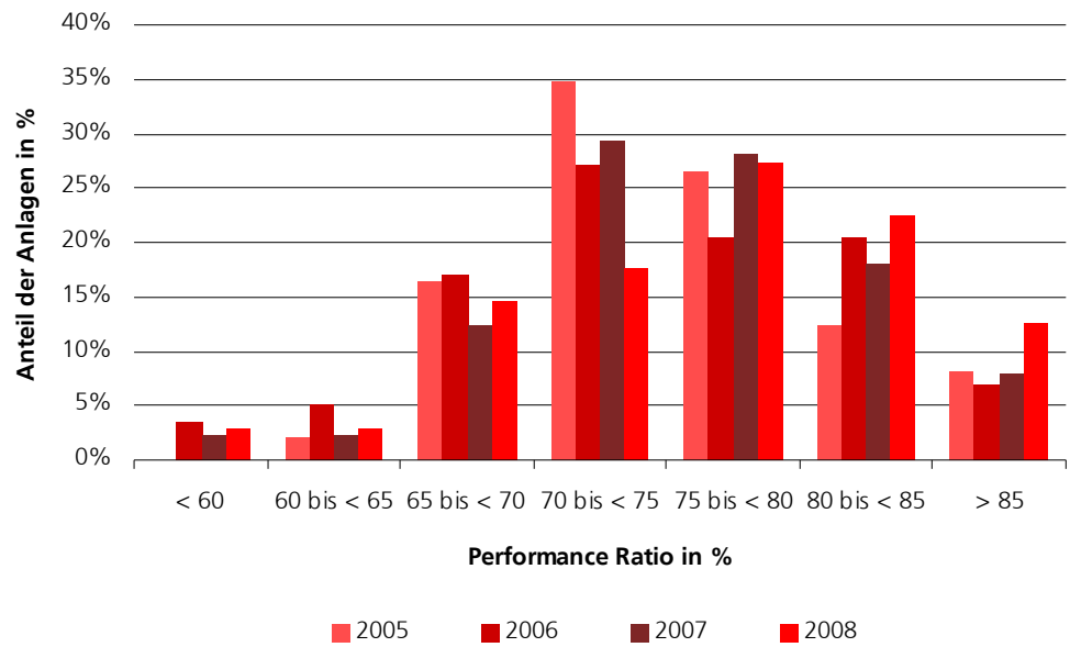
Bild 2: Verteilung der Performance Ratio für die Jahre 2005-2008
